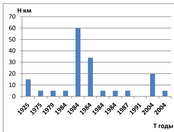
Рисунок 3. Распределение по глубине гипоцентров землетрясений в Западном Узбекистане. Долгота \lambda=62^\circ-63^\circ
