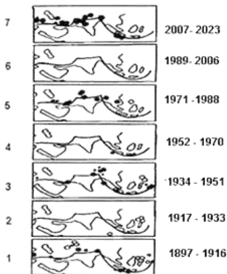
Рисунок 2. Особенности проявления сейсмичности в Азиатской части Средиземноморско-Азиатского сейсмического пояса (до 1970 г. по [К. Моги, 1974]; с 1971 г. по [К.Н. Абдуллабеков, М.Т. Усманова, 2003, 2008, 2016])
