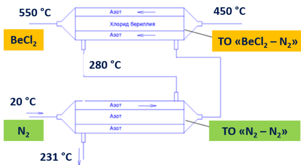
а) схема ожигения хлорида бериллия
